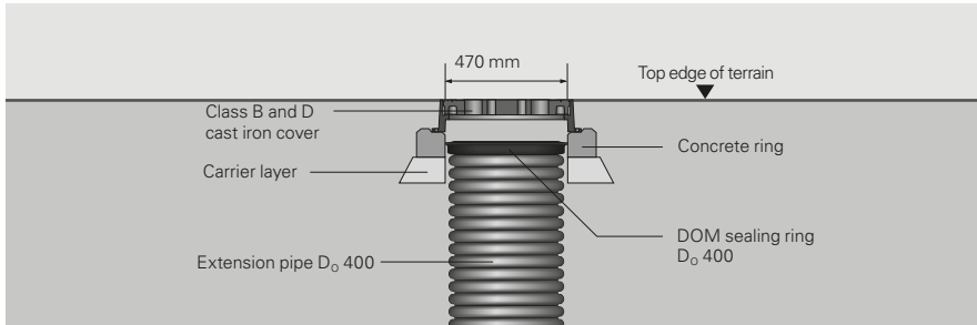
FRÄNKISCHE cover (470 mm)
